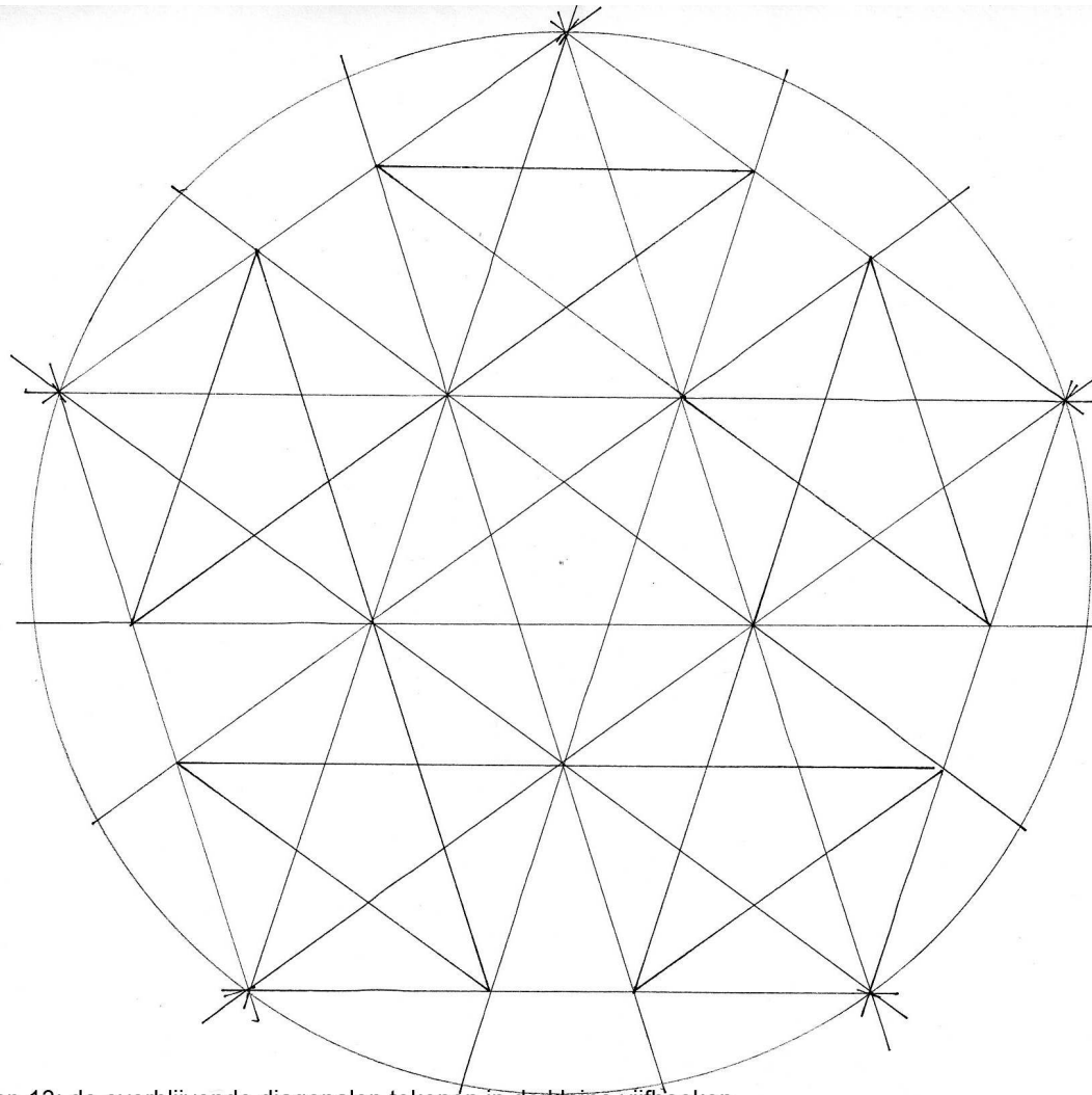
DODECAËDER stap 13: de overblijvende diagonalen tekenen in de kleine vijfhoeken.
