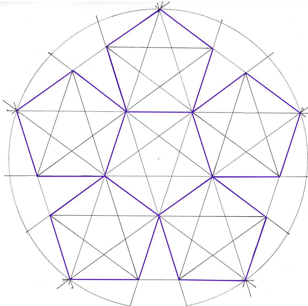
DODECAËDER stap 14: 6 vijfhoeken vormen de helft van de dodecaëder.
