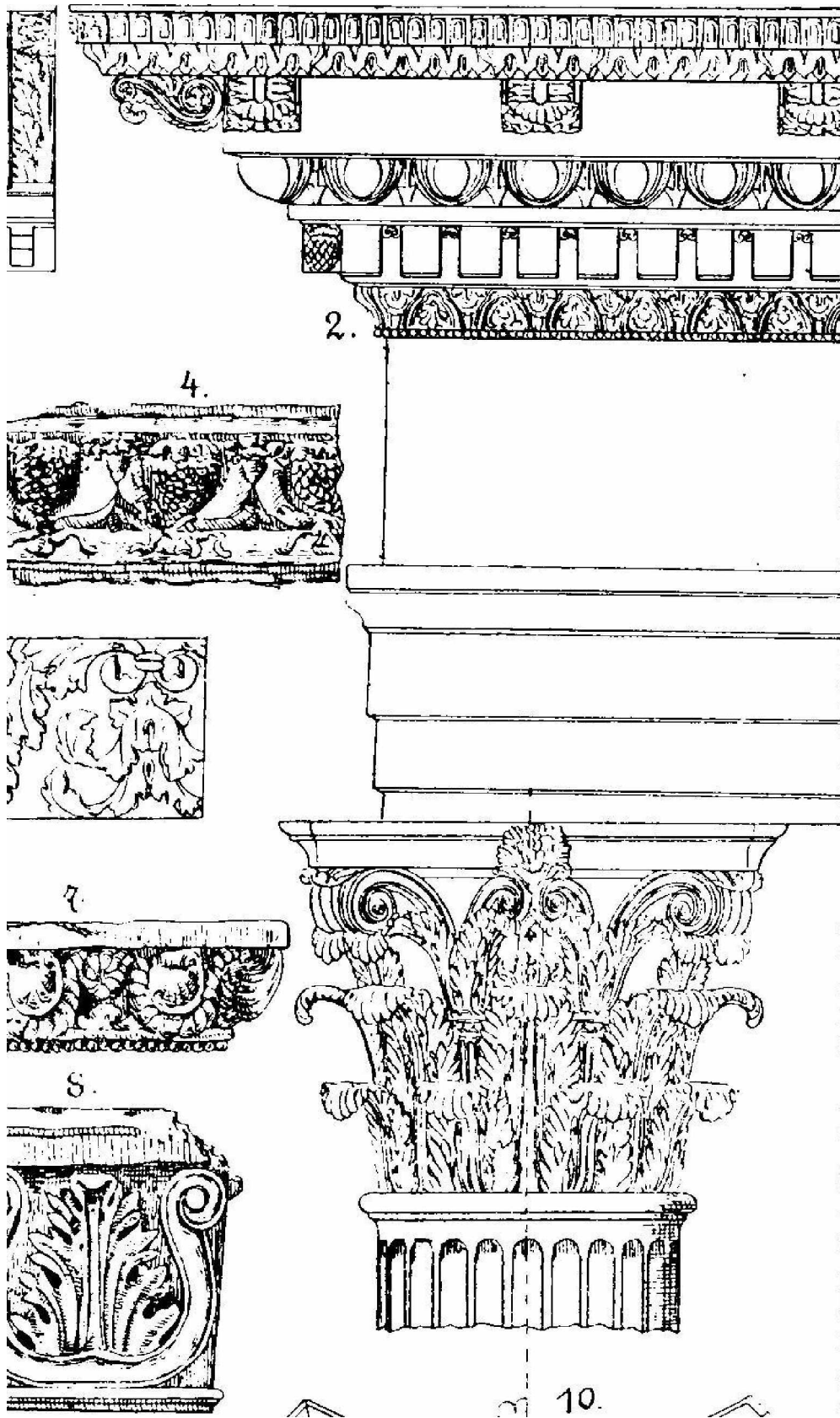
Griekenland en Rome: Korintisch Pantheon Rome
